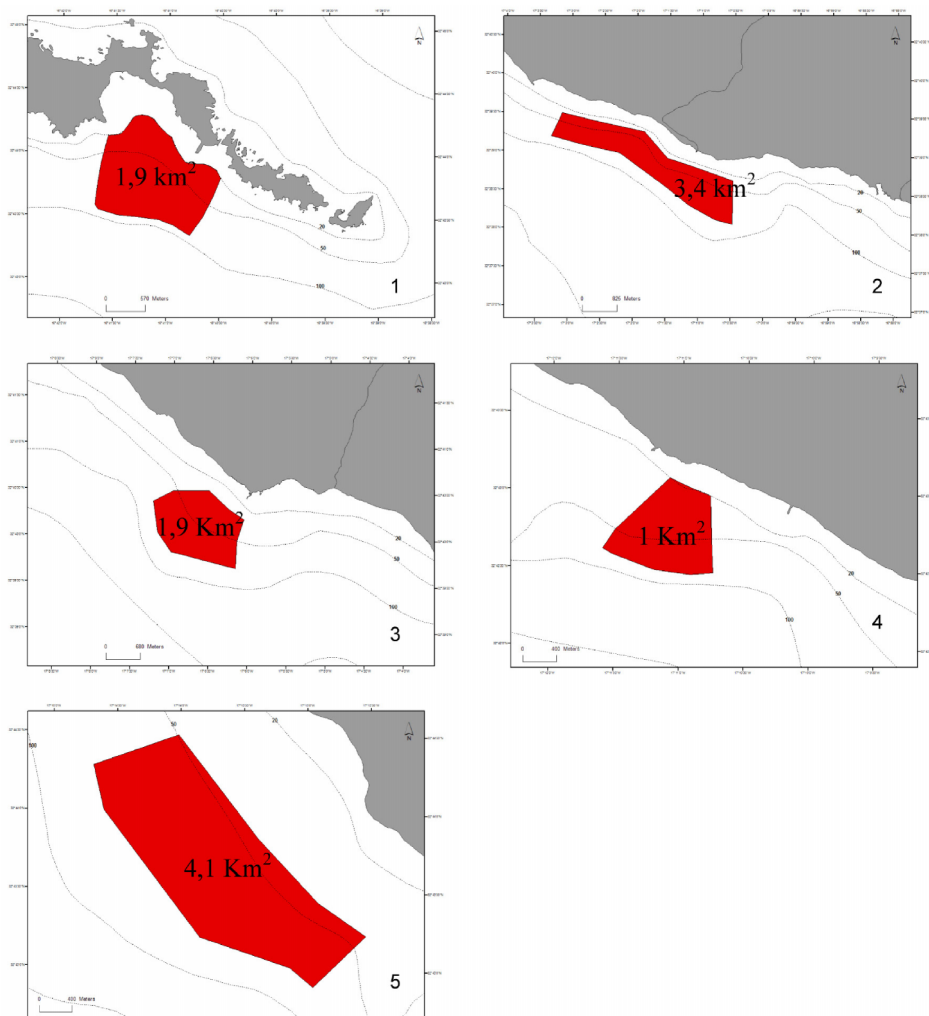
Figura 5 – Áreas selecionadas (km²) no estudo para a costa sul da ilha da Madeira. 1) Baía d'Abra; 2) eixo Cabo Girão- Ribeira Brava; 3) Anjos; 4) Ponta da Galé e 5) eixo Jardim do Mar – Paul do Mar.
