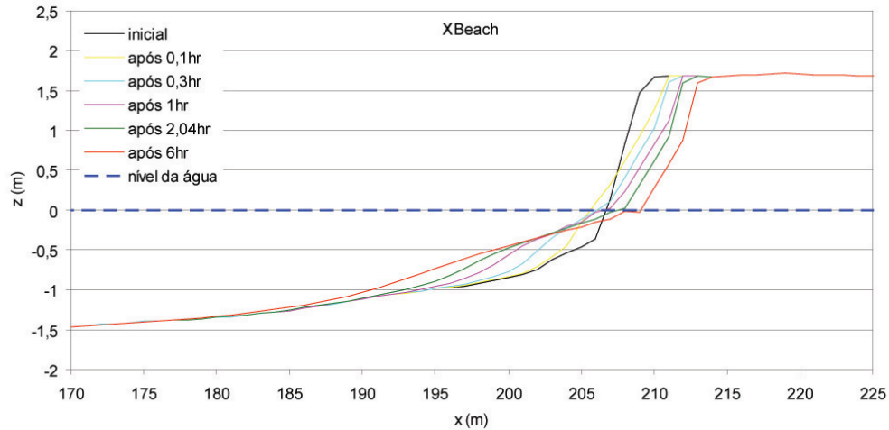
Figura 3. Resultados numéricos do modelo XBeach com parâmetros por defeito à escala laboratorial. Figure 3. Numerical results of the Xbeach model with the default parameters at laboratory scale.
