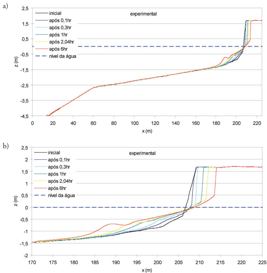
Figura 2. Evolução do perfil para o caso de verificação: a) perfil completo e b) pormenor. Figure 2. Profile evolution for the verification case: a) complete profile and b) detail.
