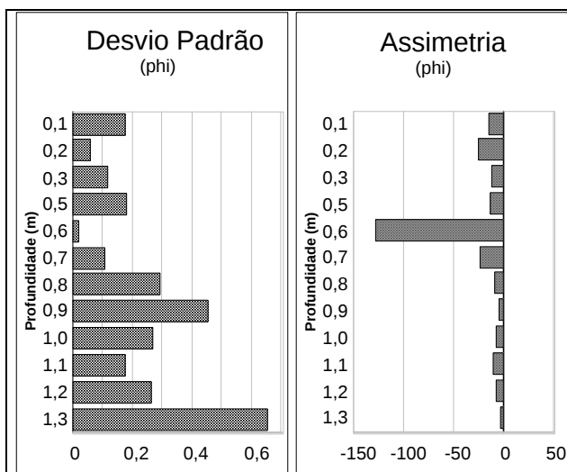
Figuras 5 e 6. Variação vertical de parâmetros estatísticos da distribuição granulométrica ao longo do perfil do Córrego dos Cadetes: 5 (esquerda): desvio padrão; 6: assimetria.
