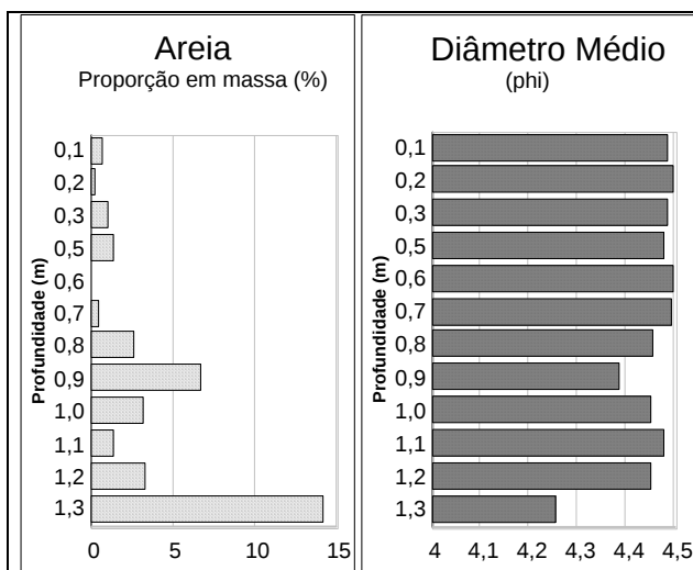
Figuras 3 e 4. Variação vertical de propriedades granulométricas ao longo do perfil do Córrego dos Cadetes: 3 (esquerda): concentração de areia; 4: diâmetro médio.
