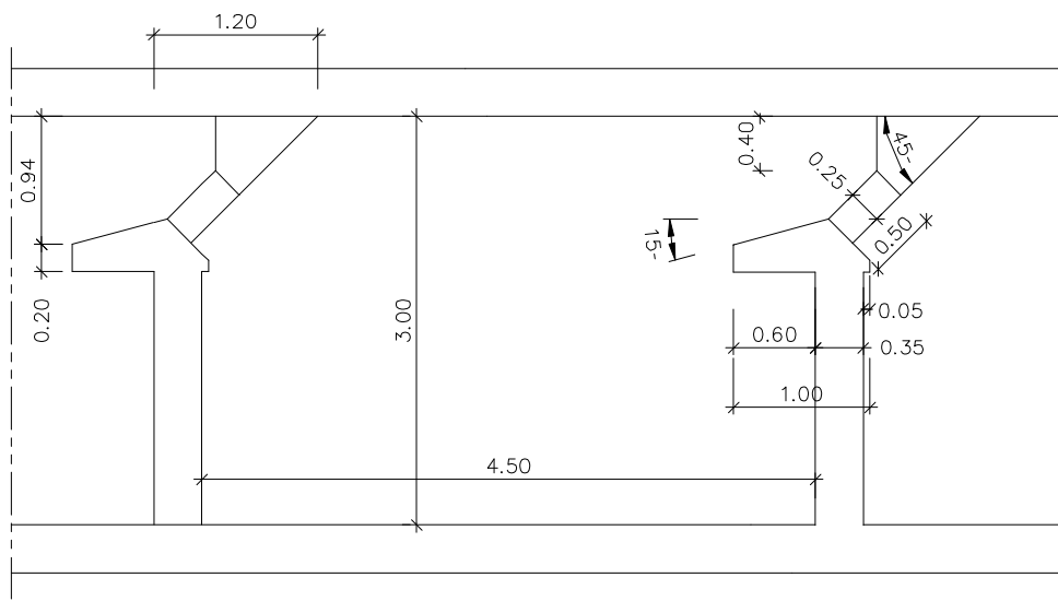
Figura 3 – Características geométricas das bacias da passagem de peixes
