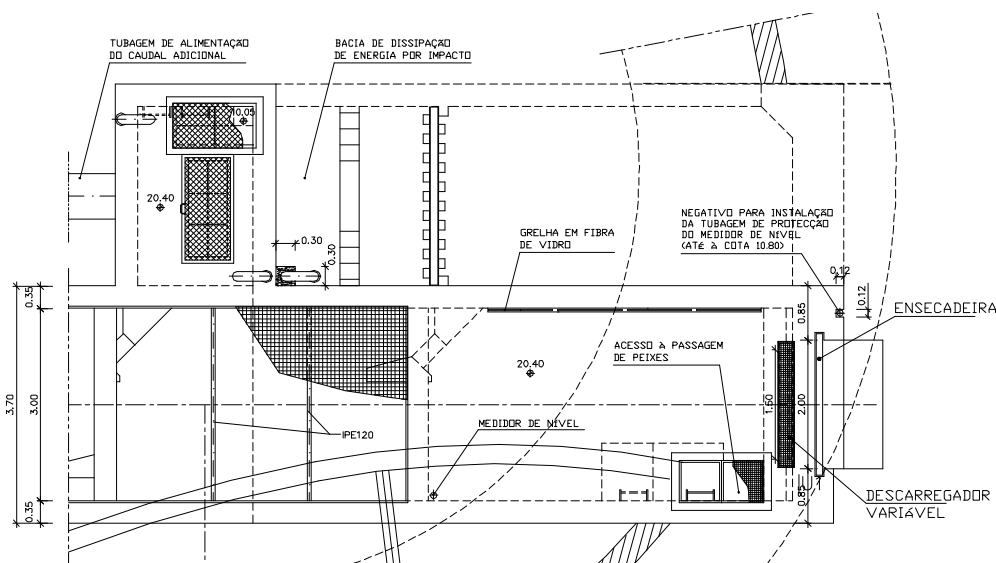
Figura 4 – Planta de cobertura da estrutura de entrada da passagem de peixes (jusante)
