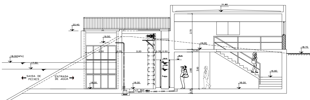
Figura 7 – Edifício de monitorização biológica e hidráulica
