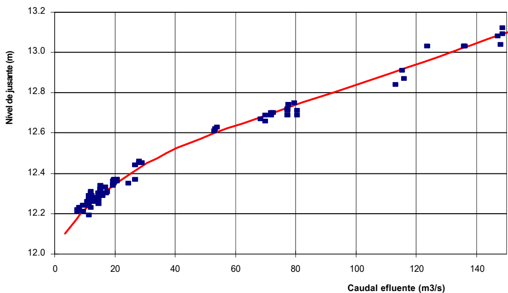
Figura 1 – Curva de vazão a jusante do Açude-Ponte de Coimbra ( Q < 150\text{m}^3/\text{s} )
