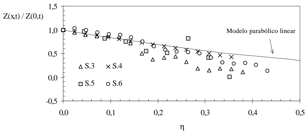
Figura 5 - Perfis longitudinais do fundo adimensionais obtidos para os ensaios S.3 a S.6.
