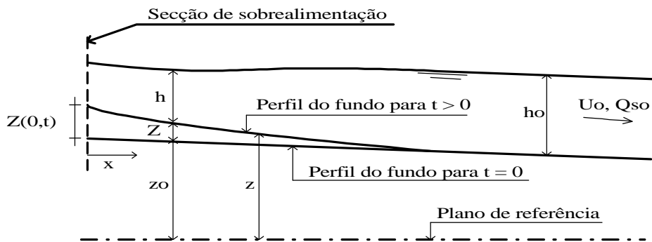
Figura 1 - Deposição devida a sobrealimentação de sedimentos. Esquema de definição.
