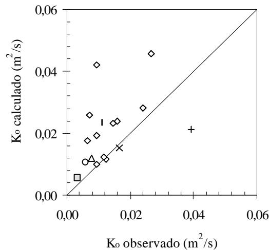
Figura 8 - Comparação entre valores observados de K_o e as previsões de Jain.
