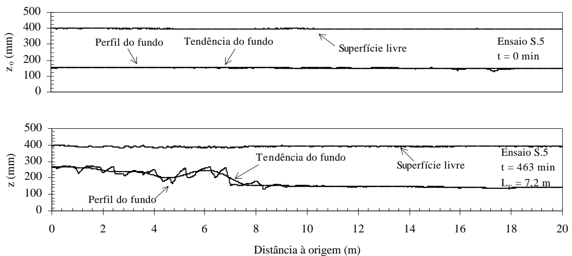
Figura 4 - Perfis longitudinais e tendências do fundo no início e no final do ensaio S.5.
