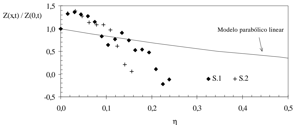
Figura 6 - Perfis longitudinais do fundo adimensionais obtidos para os ensaios S.1 e S.2.
