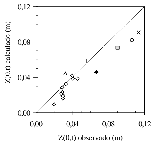
Figura 7 - Comparação entre valores observados e calculados de Z(0,t) .
