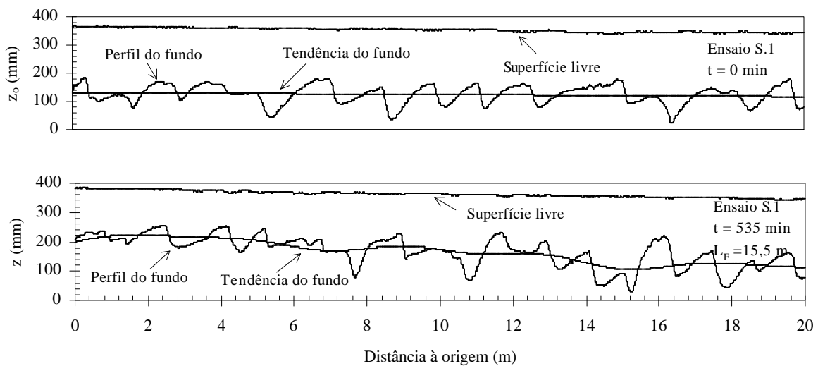
Figura 3 - Perfis longitudinais e tendências do fundo no início e no final do ensaio S.1.
