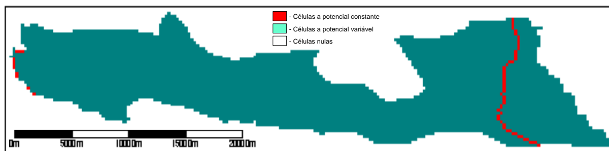
Figura 3 - Localização dos diferentes tipos de células incluídas na malha do modelo.
