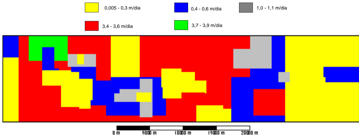
Figura 7 - Projecção das condutividades hidráulicas horizontais na malha do modelo. As zonas correspondentes às células inativas não têm qualquer significado.
