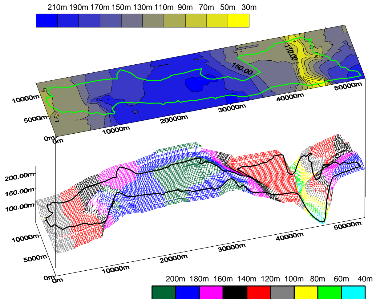
Figura 9 - Duas perspectivas da distribuição dos níveis calculados pelo modelo de escoamento: a superior a duas dimensões e a inferior a três dimensões. Os sectores externos aos contornos (verde e preto) não têm qualquer significado.
