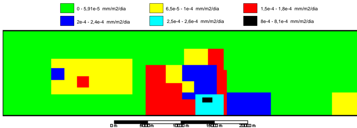
Figura 8 - Distribuição da recarga na malha do modelo. As zonas correspondentes às células inativas não têm qualquer significado.
