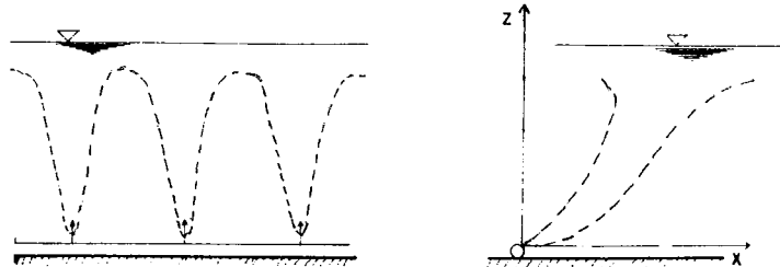
Fig.3- Sistema de jactos múltiplos submersos
