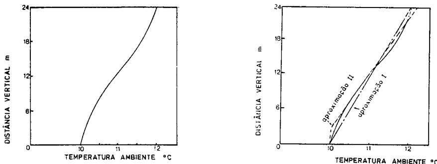
Fig.5 - Perfil de temperaturas e aproximações consideradas.
