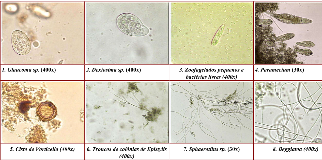
Figura 3 (3.1 – 3.4) Indicadores para sobrecarga das estações de tipo aeração prolongada :
