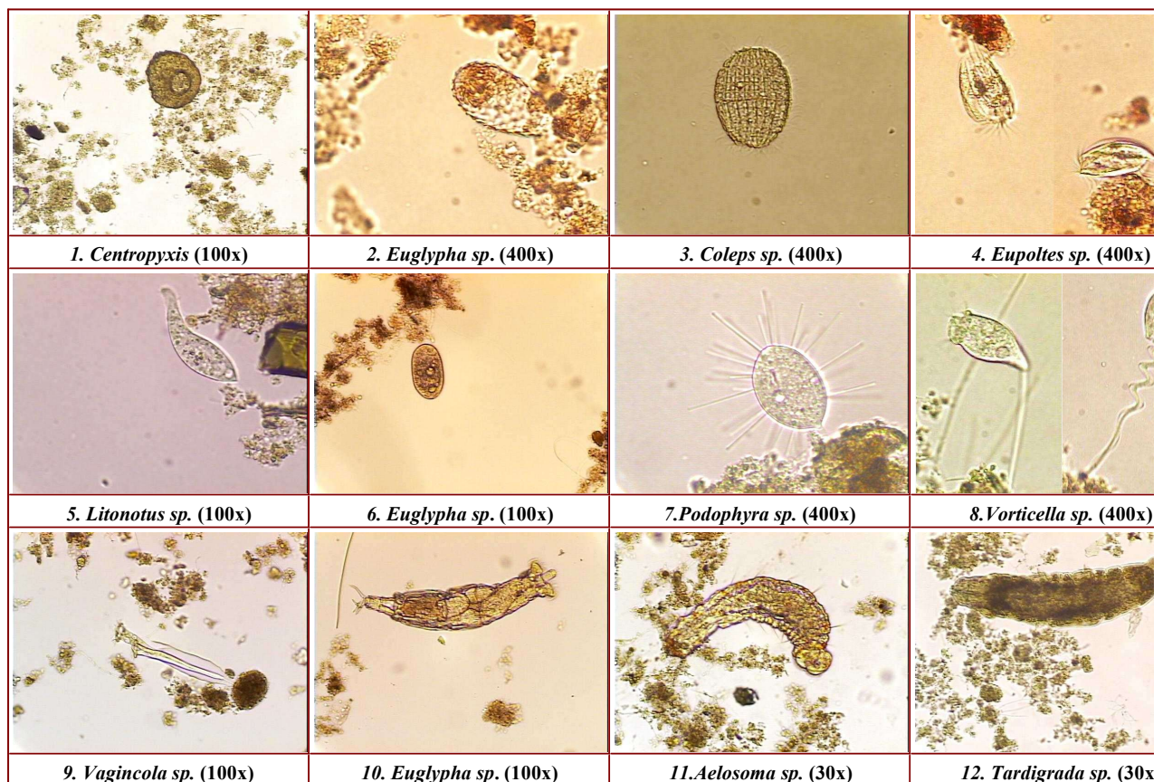
Figura 1 (1.1 – 1.12) Indicadores para alta idade de lodo e operação estável:
