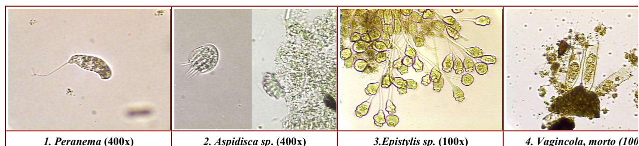
Figura 2 (2.1 – 2.4) Indicadores para a sobrecarga das estações de tipo aeração prolongada :
